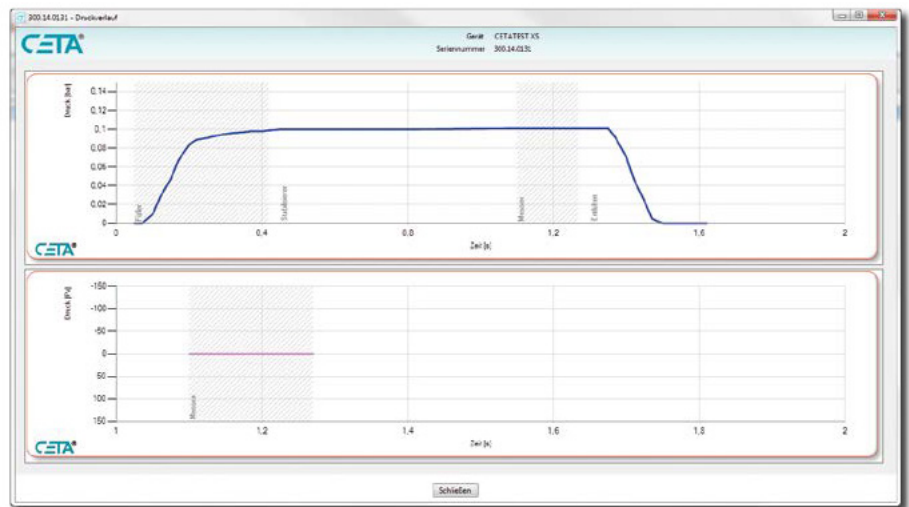
Darstellung der Druckverlaufskurve
